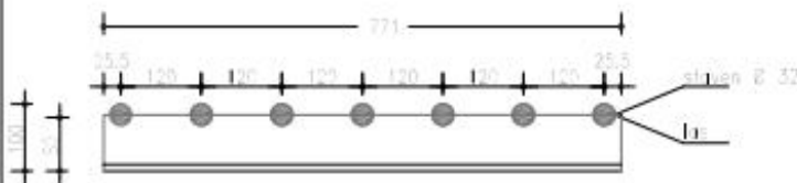
Aanzicht L 80.80.10
