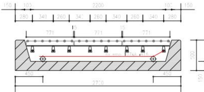
Dwarsdoorsnede
